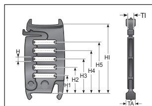
Полочный держатель
